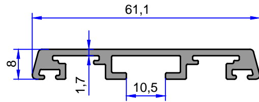
4942 0.576 kg/m
