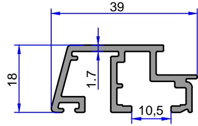
4445 0.494 kg/m
