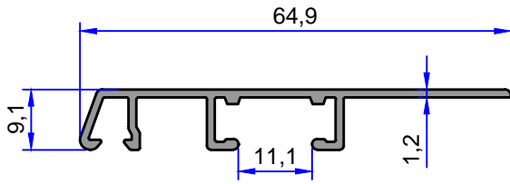
5865 0.351 kg/m
