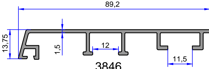
3846 0.667 kg/m
