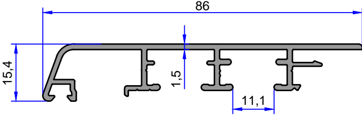
5866 0.685 kg/m
