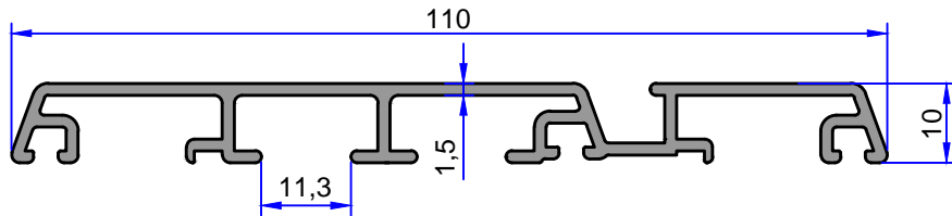
5453 0.866 kg/m
