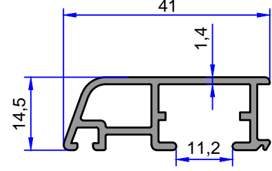
5452 0.416 kg/m
