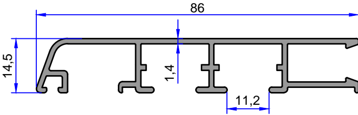
5451 0.737 kg/m
